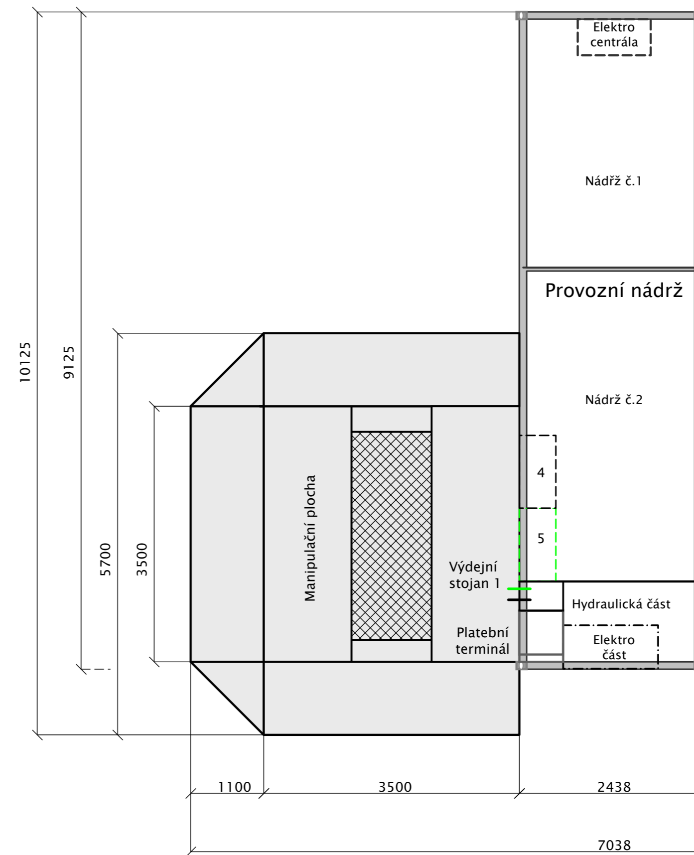
Půdorys (řez A-A)
